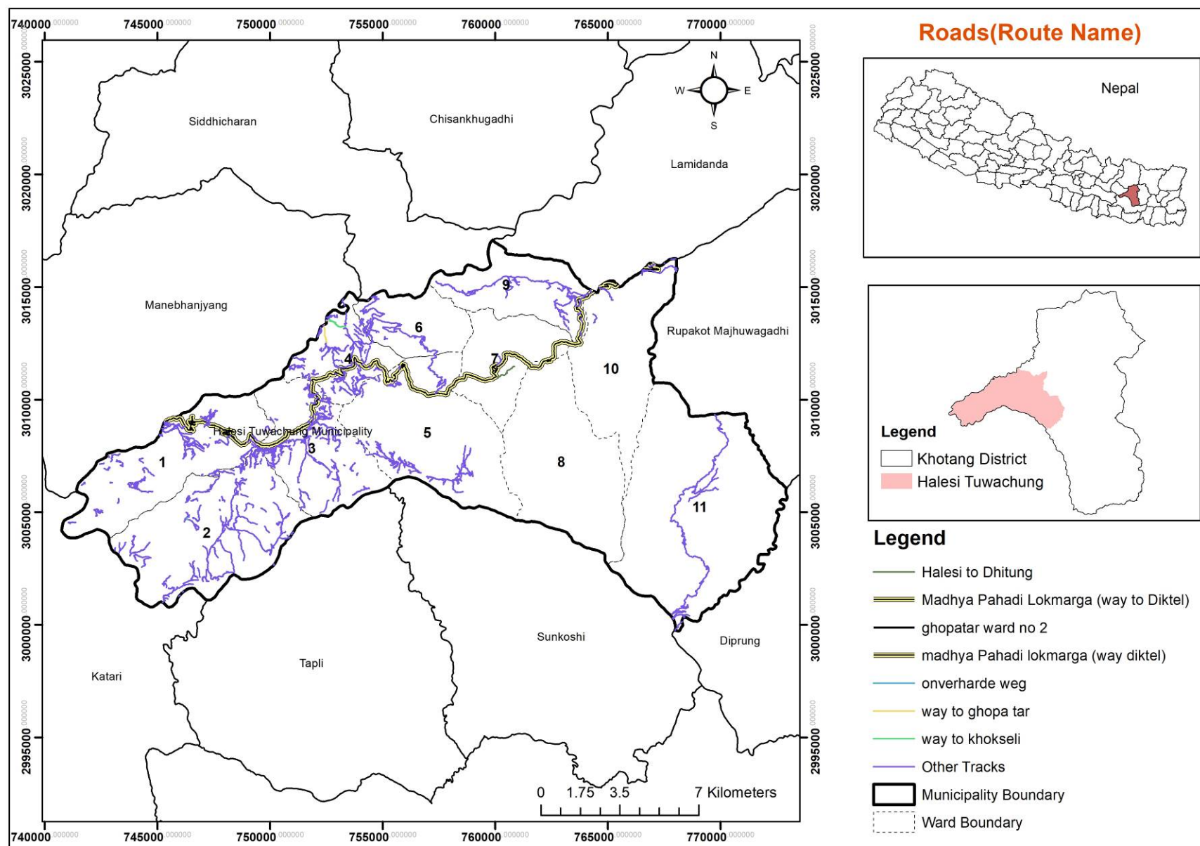
चित्र ११: हलेसी तुवाचुङ नगरपालिकाको सडक संजाल (बाटोको नाम सहित)
